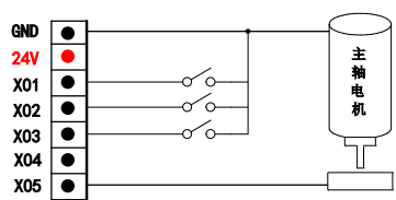
机械回零开关接线图
