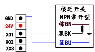
光电回零开关接线图
