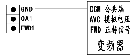
变频器接线图-模拟量
